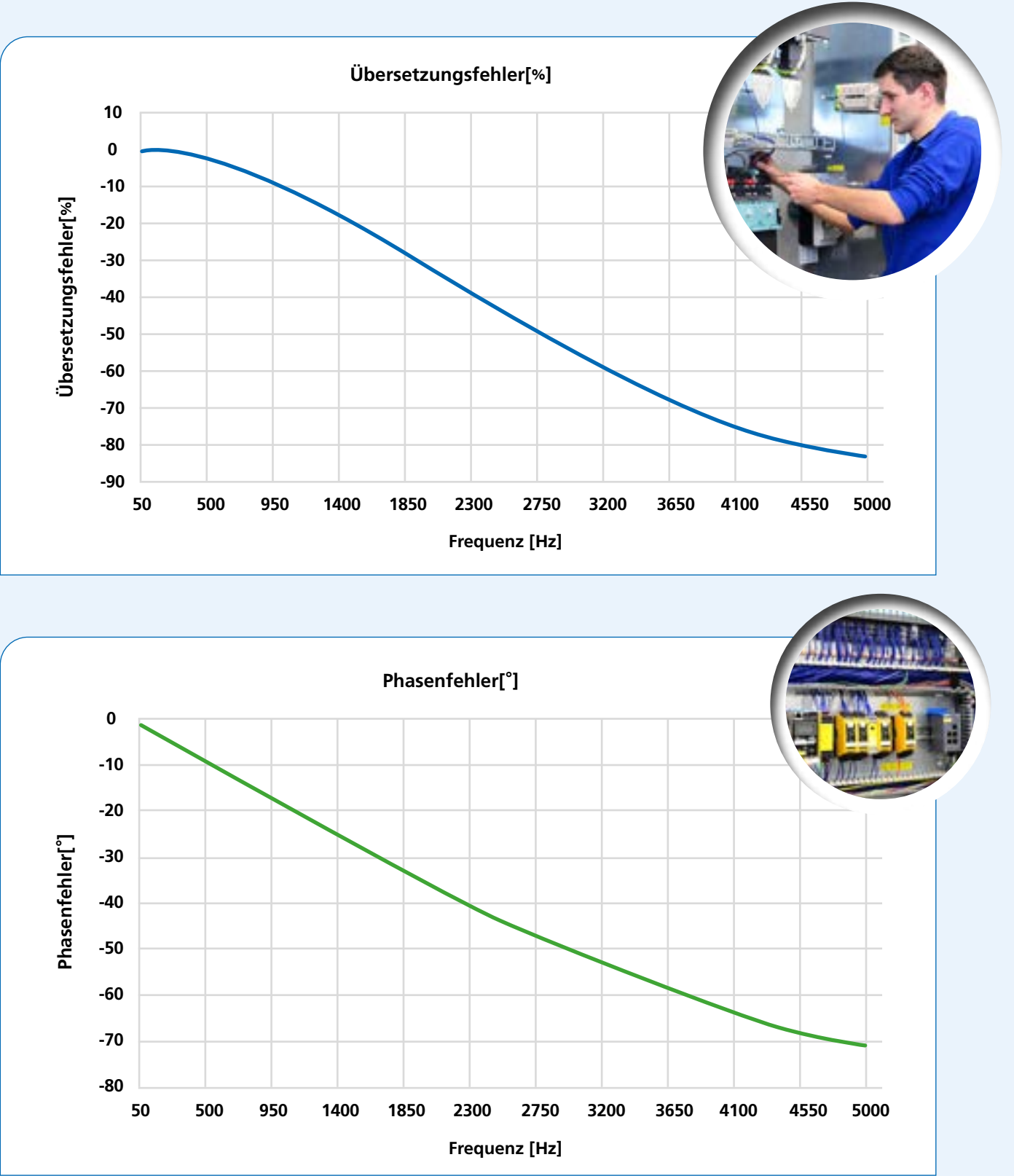
Abbildung 11: Frequenzübertragungsverhalten des ROI-3 mit einer FASK 150 (Amplitudenfehler und Phasenfehler)
