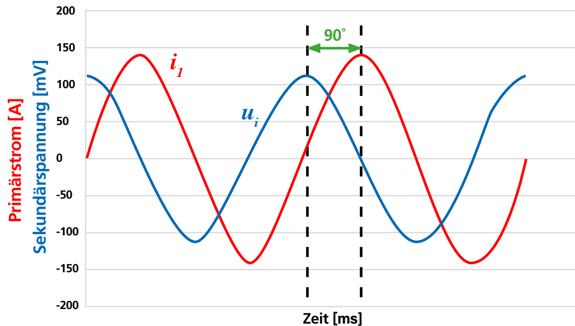
Abbildung 2: Primärstrom und Ausgangssignal einer passiven Rogowski-Spule im Vergleich
