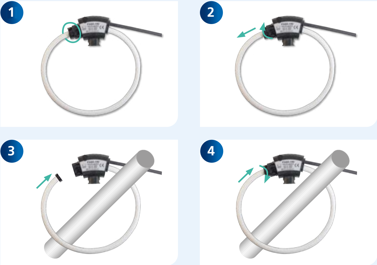
Abbildung 6: Montage der FASK
