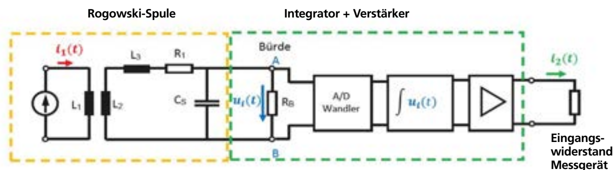
Abbildung 3: Elektrisches Ersatzschaltbild Rogowski-Spule + 1 A Integrator
