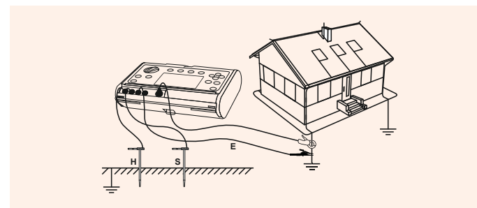
Messen des Erdungswiderstandes - 3-Pol-Methode + Zange
