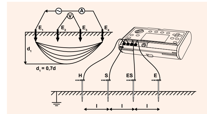
Messung des spezifischen Erdwiderstands nach der Wenner-Methode
