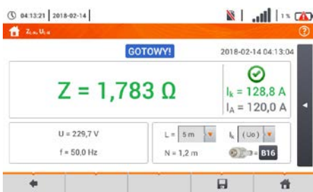
Fehlerschleifenimpedanzmessung
