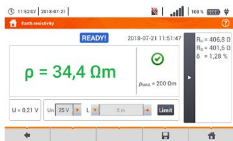
Messen des spezifischen Erdwiderstandes
