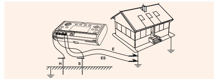
Messen des Erdungswiderstandes - 4-Leiter-Methode
