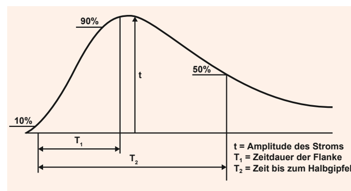
Form des Messimpulses bei der Impulsmethode
