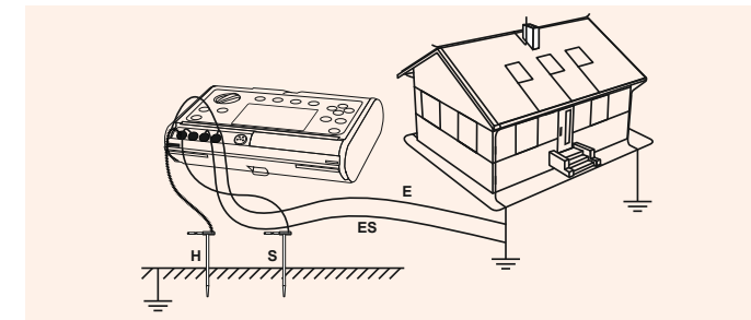
Erd-Impedanzmessung (4p-Impulsmethode)
