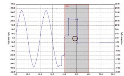
Beispiel eines Stromausfalls (Blackout)
