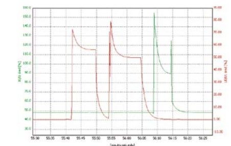
Beispiel für eine durch eine Verbindung hervorgerufene Asymmetrie
