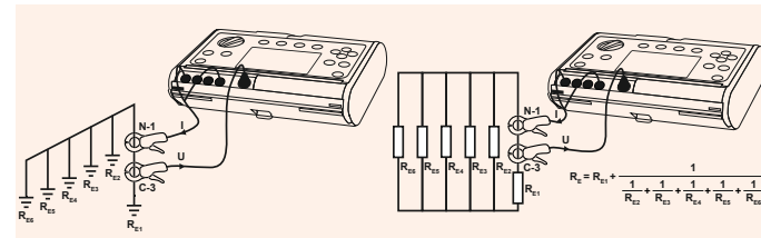
Anschlussart des Messgeräts bei der 2-Zangen-Methode
