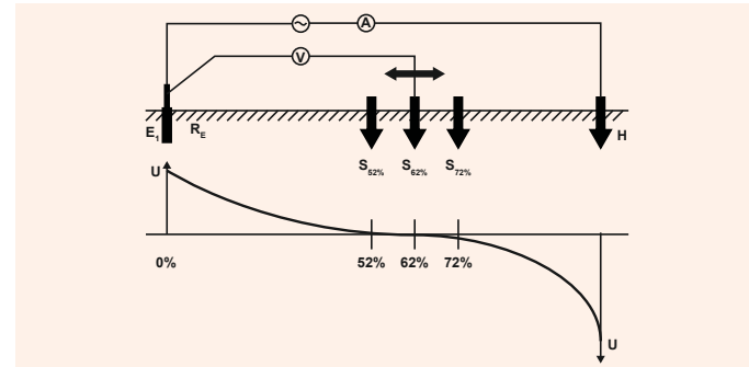
Spannungsverteilung während der Messung
